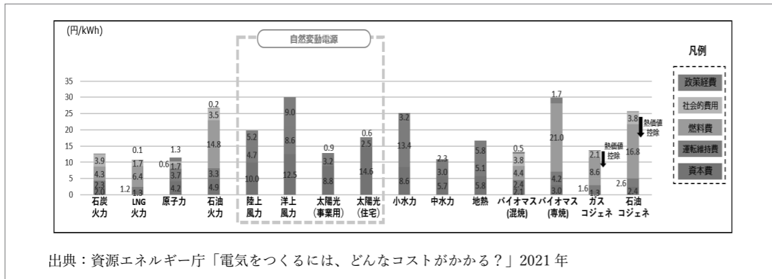
【資料7】2020年の国内電源別発電コスト
